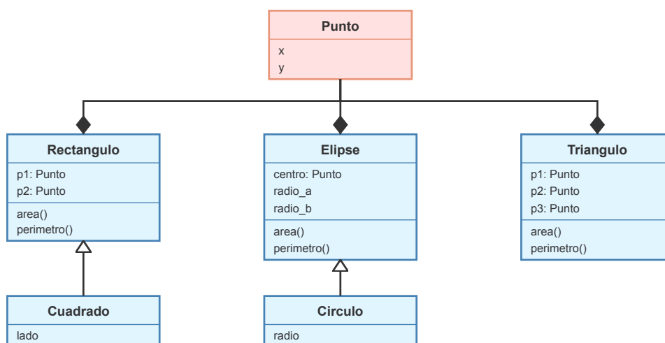
Figure 1.8: Diagrama de clases de Figuras Geométricas
