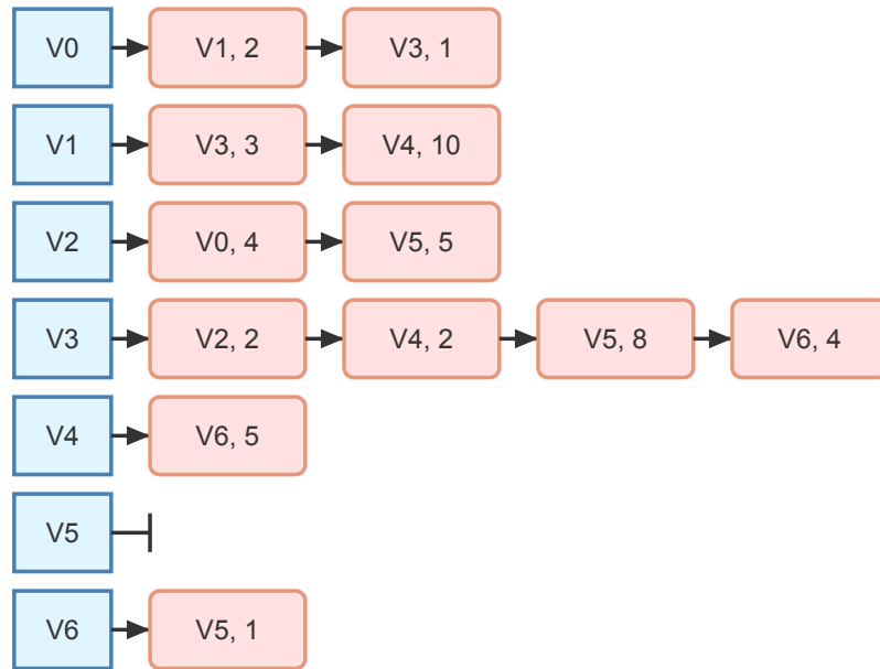
Figure 2.13: Lista de adyacencia del grafo dirigido
