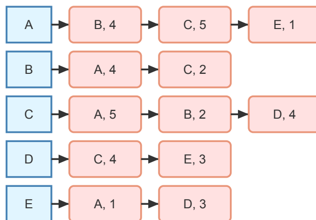
Figure 2.14: Lista de adyacencia del grafo no dirigido
