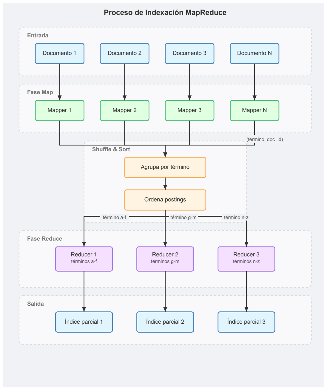
Figure 4.4: Indexado con Map-Reduce
