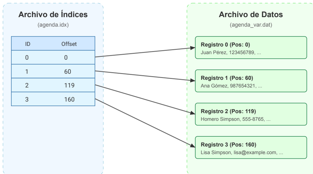
Figure 3.1: Archivo de índices
