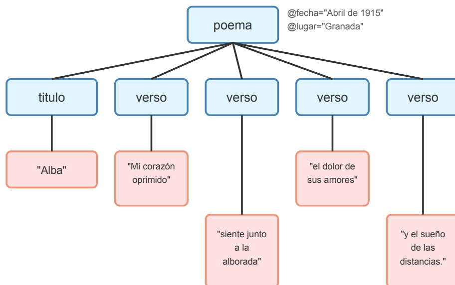
Figure 3.3: Árbol que representa la estructura del poema en XML.
