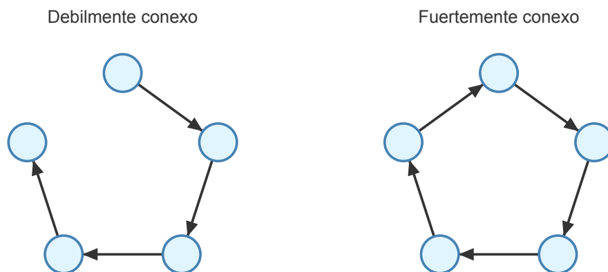
Figure 2.5: Grafos conexos dirigidos
