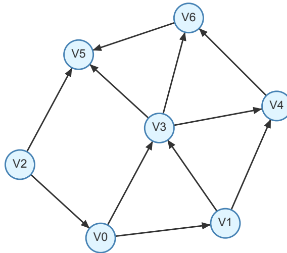
Figure 2.17: Grafo Dirigido Acíclico
