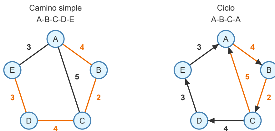
Figure 2.7: Caminos en grafos
