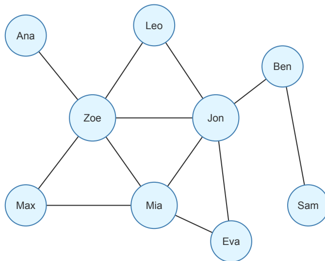
Figure 2.2: Grafo de amistades en una red social
