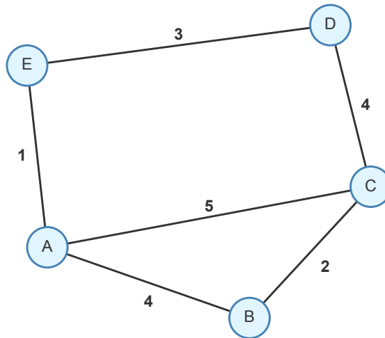
Figure 2.6: Grafo ponderado con costos en las aristas
