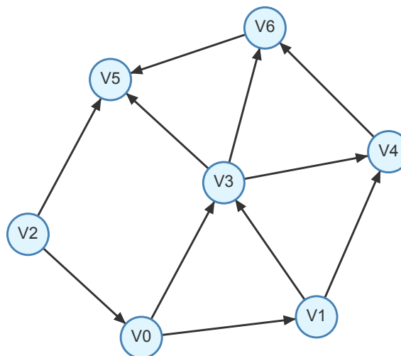
Figure 2.8: Grafo Dirigido Acíclico
