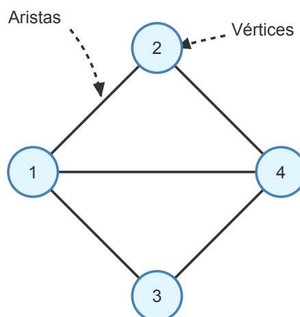
Figure 2.1: Ejemplo de un grafo
