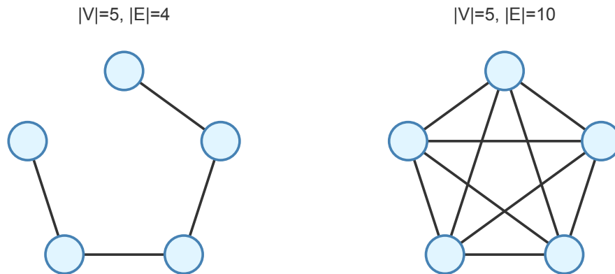
Figure 2.4: Grafos conexos no dirigidos
