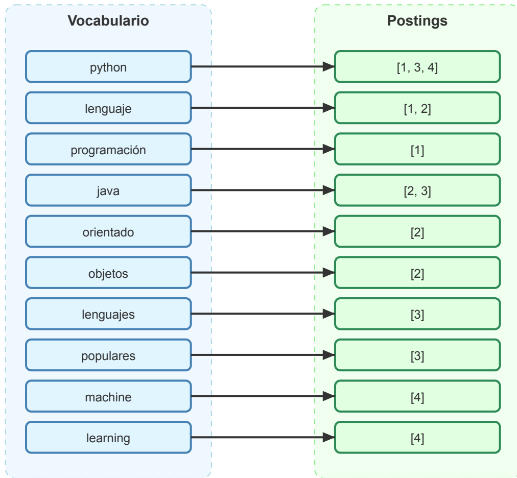
Figure 4.3: Estructura de un índice invertido
