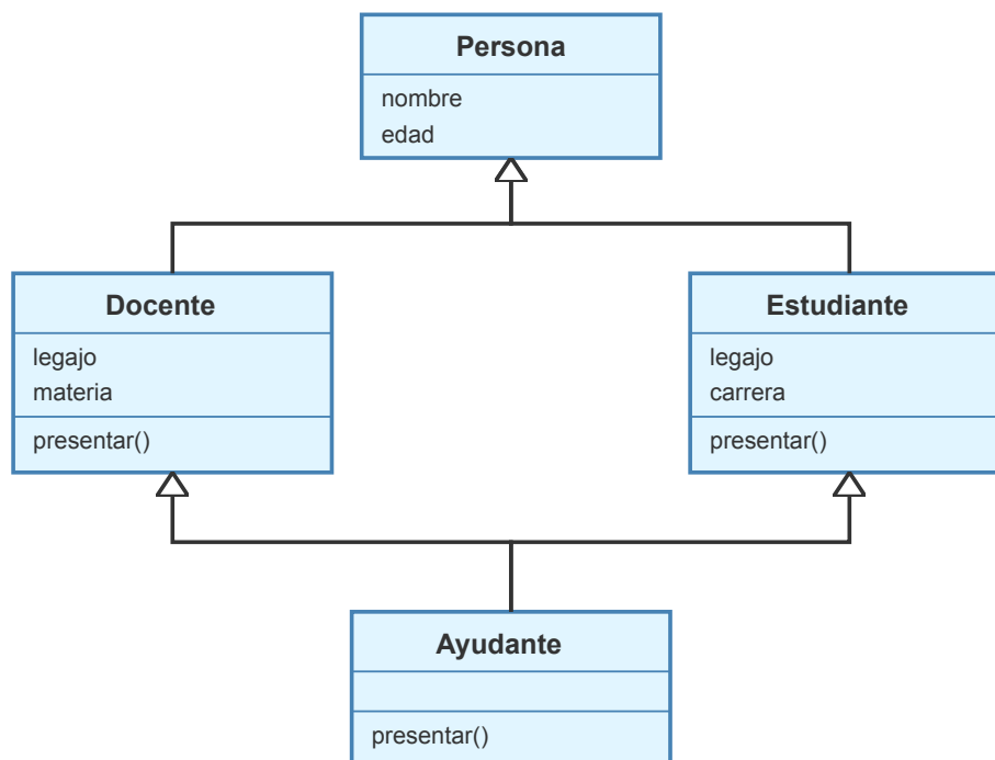
Figure 1.7: Diagrama de clases de Ayudante
