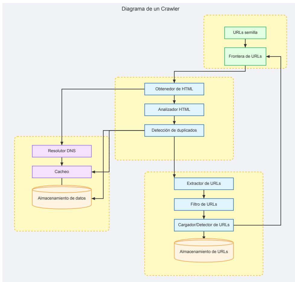
Figure 3.7: Arquitectura básica de un crawler
