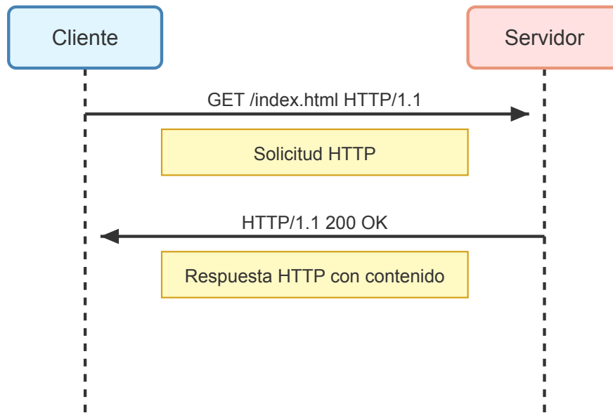
Figure 3.5: Interacción HTTP Cliente-Servidor
