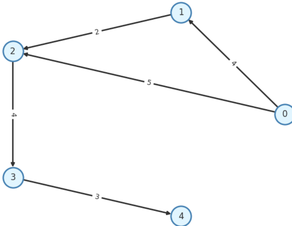
Grafo Dirigido
