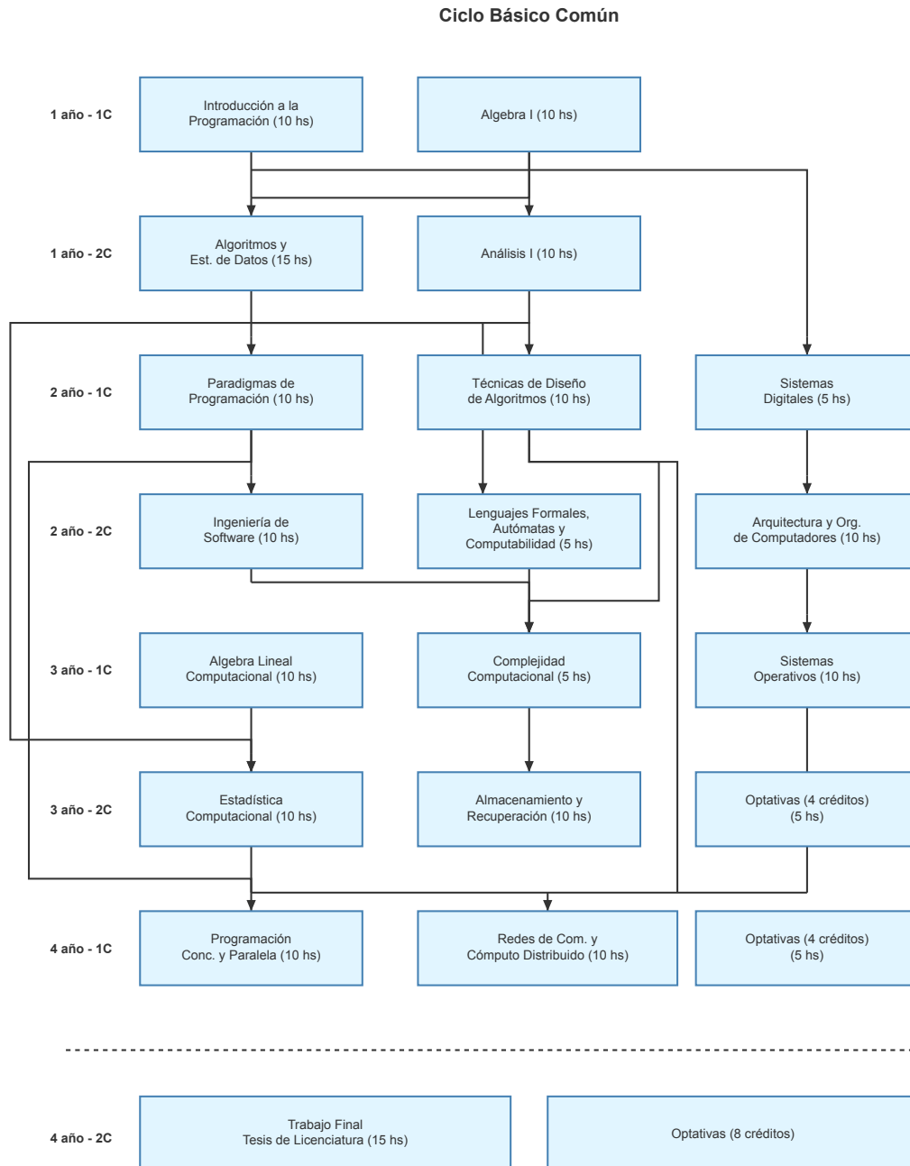
Figure 2.3: Grafo de correlativas en un plan de estudios
