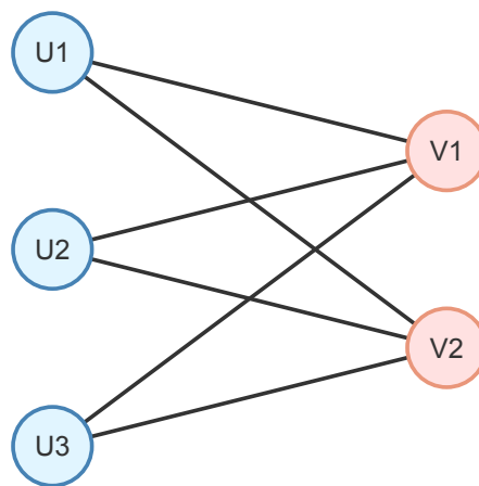
Figure 2.16: Grafo Bipartito Ordenado
